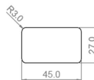
Pannello di montaggio Mounting template
